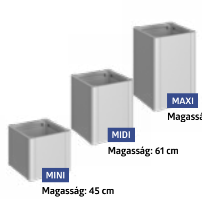
11 Magasság változatok
