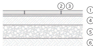
Lapok fektetése laptartó tappancsra (csak gyalogos forgalmú felületek)
