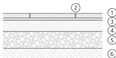
Lapok fektetése habarcságyra (gyalogos forgalmú felületek)
