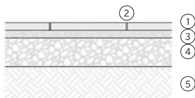
Lapok fektetése kavicságyra (csak gyalogos forgalmú felületek)
