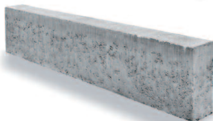
Térburkoló szegély kopóréteggel Méret: 100 x 25 x 8 cm Szín: szürke
