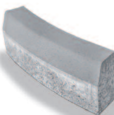
Íves útszegélyek Méretek: 39 x 25 x 15 cm, R = 0,5 m 52 x 25 x 15 cm, R = 1,0 m 78 x 25 x 15 cm, R = 2,0 m 78 x 25 x 15 cm, R = 3,0 m Szín: szürke
