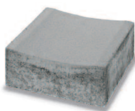
Betonfolyóka 1,5 cm horonymélységgel Méret: 40 x 40 x 8 cm Szín: szürke
