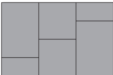
Citytop Grande Kombi rakatkép 20 x 40 x 6 cm: 2 db 40 x 40 x 6 cm: 2 db 60 x 40 x 6 cm: 2 db
