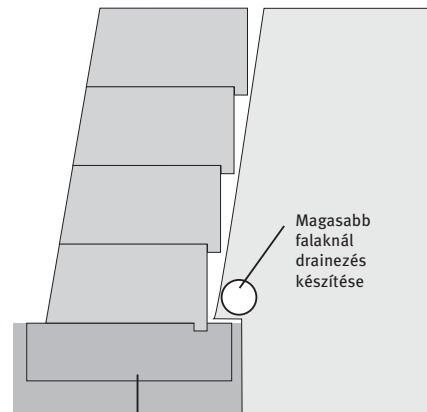
Megfelelő beton alaptést készítése
